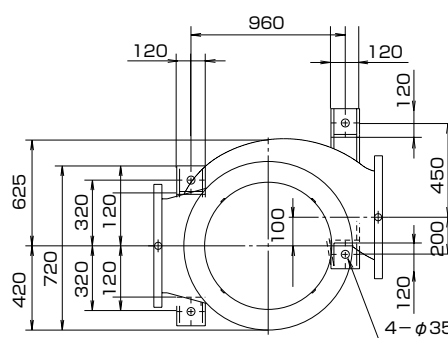
ESD-450C
