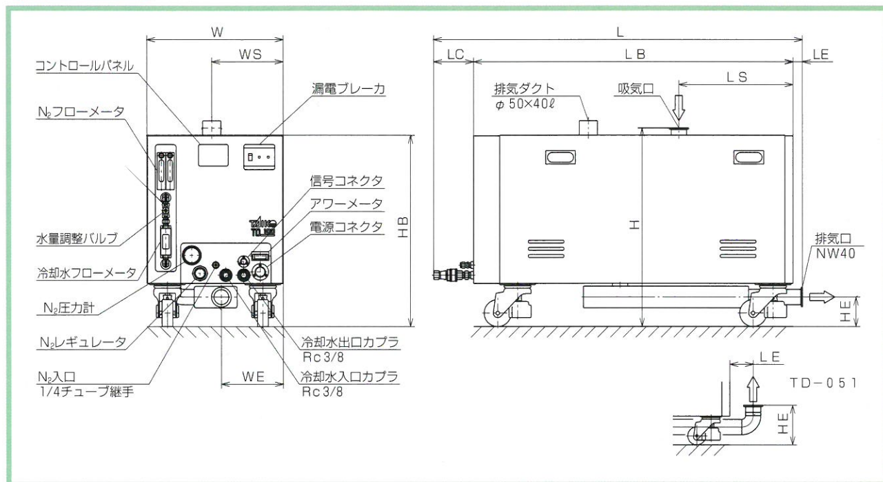
寸法表(mm)
